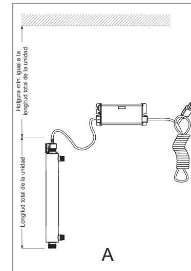
Figura 3 Instalación del sistema de desinfección: vertical y horizontal
